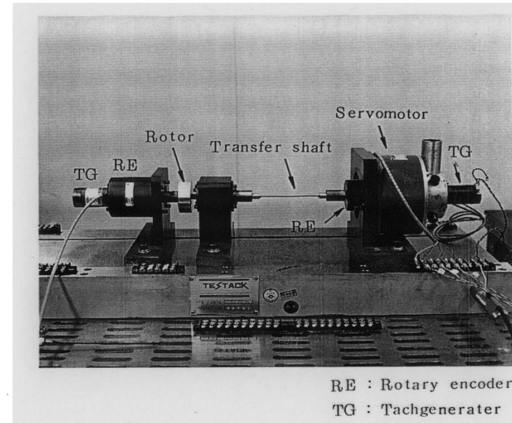
負荷系の振動特性を模擬した サーボモータ系の実験装置
