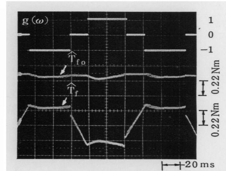
適応外乱オブザーバ
