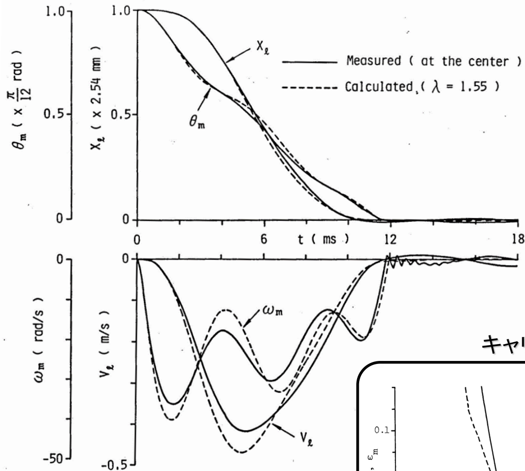
3設定値系による位置決め制御 ( T=12\text{ms} )
