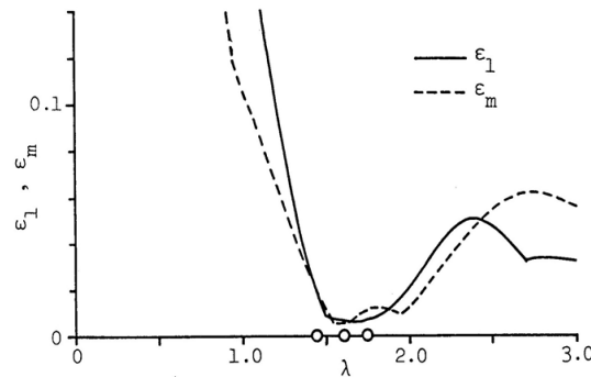
(a) 3設定値系 ( \lambda_0=1.45, 1.60, 1.75 )
