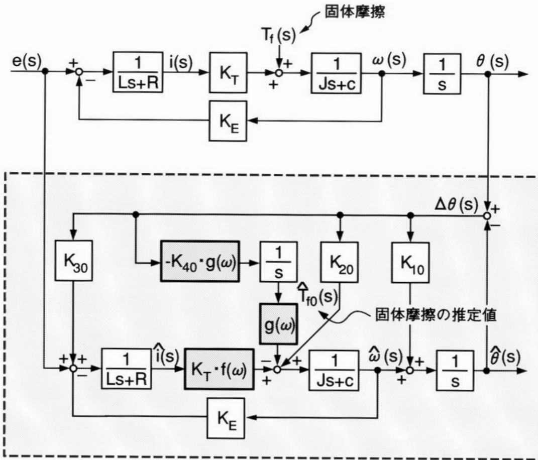
適応外乱オブザーバのブロック図
