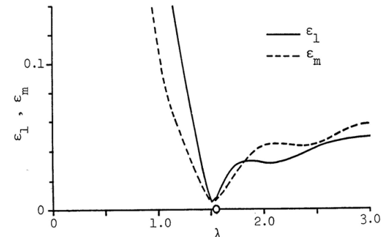
(b) 1設定値系 ( \lambda_0=1.55 )
