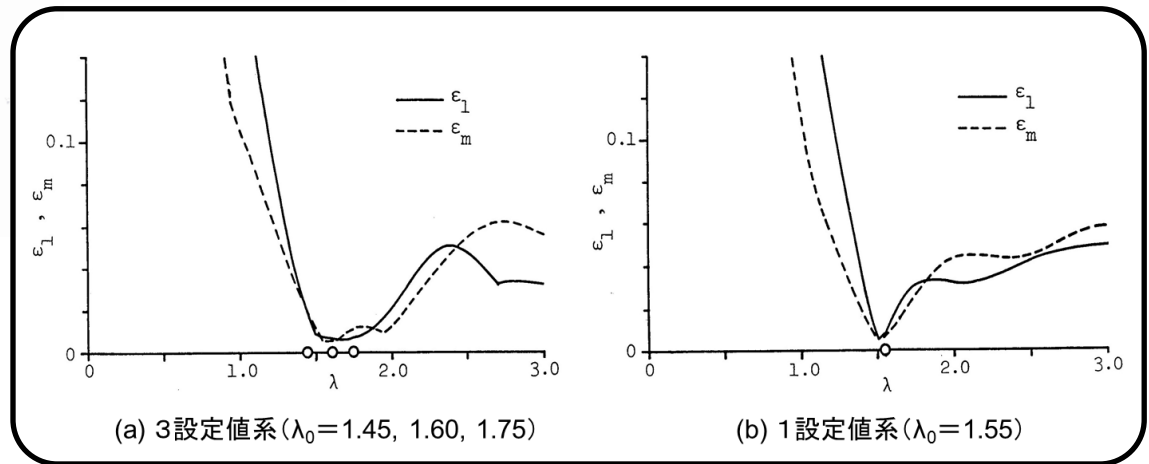
3設定値系による位置決め制御 ( T=12\text{ms} )
